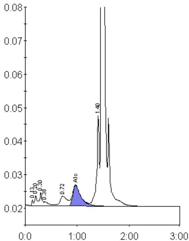
Peak table - ID: 60001211
